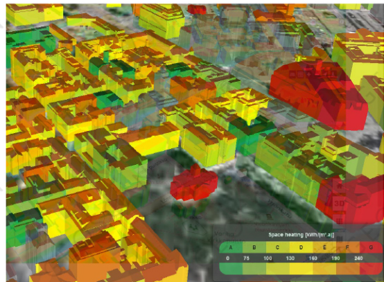
Карта энергопотребления
